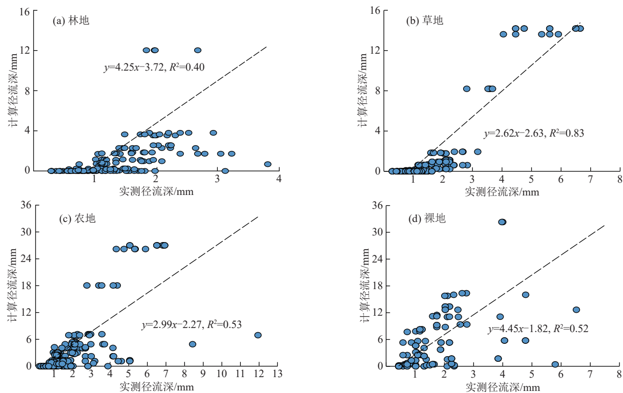
图 1 标准 SCS-CN 法的径流模拟 Fig. 1 Runoff simulation with standard SCS-CN
